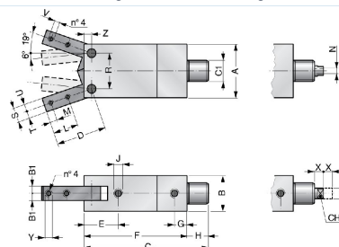
Version durchgehende Kolbenstange:
