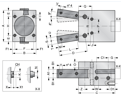
Version durchgehende Kolbenstange
