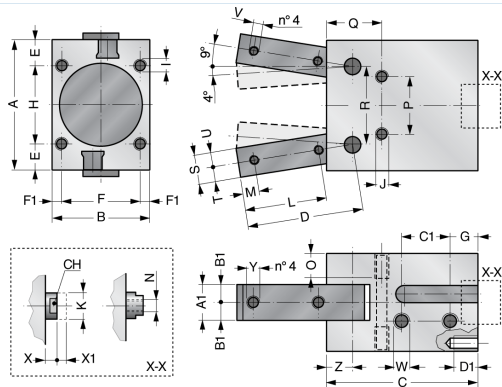
Kivitel átmenő dugattyúrúd
