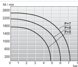
Průtokový diagramm 1/4"
