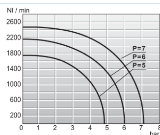
Wykres przepływu 1/4"
