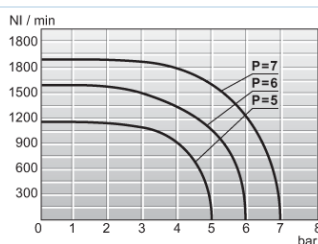
Átfolyási diagramm 1/4"
