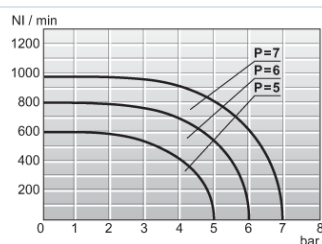
Átfolyási diagramm 1/8"
