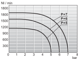
Wykres przepływu 1/4"
