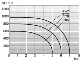
Wykres przepływu 1/8"
