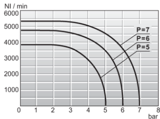
Wykres przepływu 1/2"
