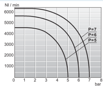
Wykres przepływu 1/2"
