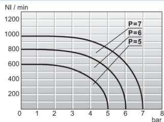
Durchflussdiagramm 1/8"
