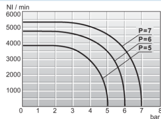
Durchflussdiagramm 1/2"
