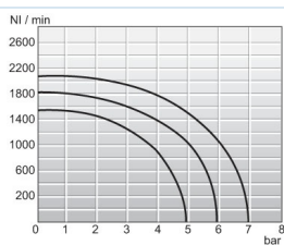
Átfolyási diagramm 1/4"
