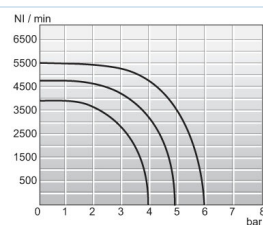
Átfolyási diagramm 1/2"
