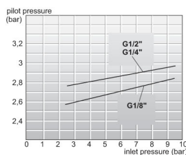
Ovládání pneumaticky/pružina
