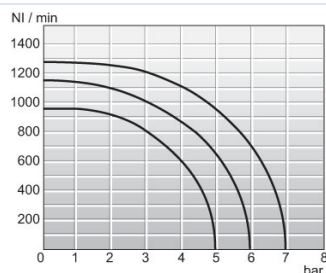
Wykres przepływu 1/8"
