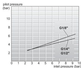
Aktiviranje pneumatski/interni upravljački vazduh
