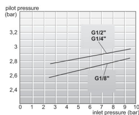
Aktiviranje pneumatski/opružno vraćanje
