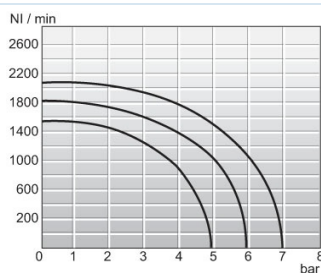
Átfolyási diagramm 1/4"
