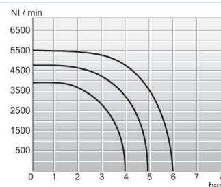
Átfolyási diagramm 1/2"
