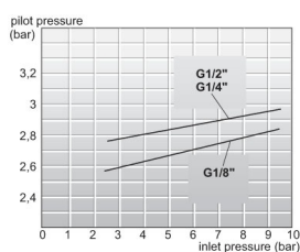
Uruchamianie pneumatyczne/sprężyna
