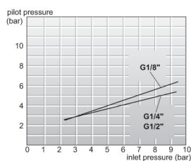
Uruchamianie pneumatyczne/wewnętrzne powietrze sterujące
