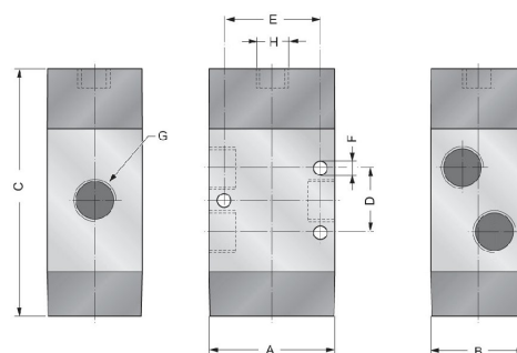
Uruchamianie pneumatyczne/wewnętrzne powietrze sterujące
