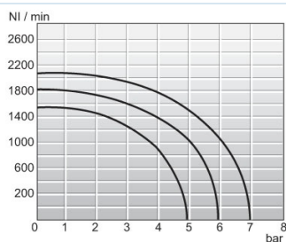
Wykres przepływu 1/4"
