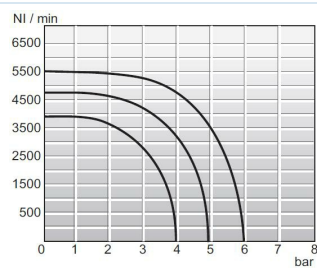
Átfolyási diagramm 1/2"
