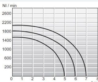
Wykres przepływu 1/4"
