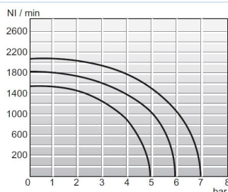
Durchflussdiagramm 1/4"
