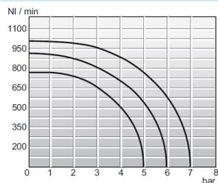
Průtokový diagramm 1/8"
