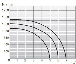
Wykres przepływu 1/4"
