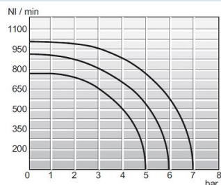
Wykres przepływu 1/8"
