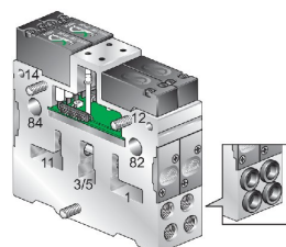
Modul für Magnetventilstation elektrisch/Feder - _ _ -
