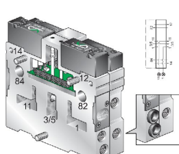
Modul Arbeitsdruckseparator - _ Y - mit Einzelstation-Modul
