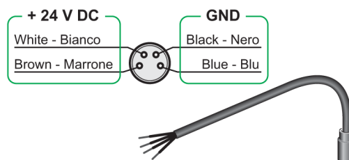
CW-PS Napájecí kabel
