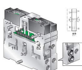
Modul separátor pracovního tlaku - Y _ - s modulem jednotlivé stanice
