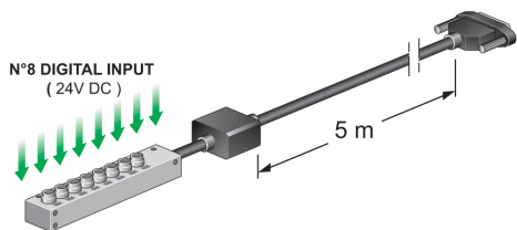
SCBI 8-M8 Doboz 8 bemenethez (24V DC)
