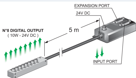
SCBO 88-M Doboz 8 digitális kimenethez (10W - 24V DC)
