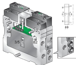
Modul Üzemi nyomásleválasztó - X _ - egydi állomásmodullal
