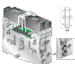
Modul Üzemi nyomásleválasztó - _ Y - egydi állomásmodullal
