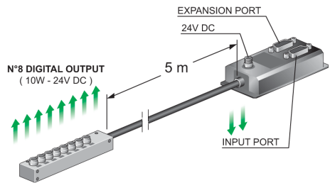
SCBO 88-M Skrzynka na 8 wyjść cyfrowych (10W - 24V DC)
