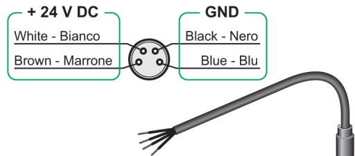
CW-PS Przewód zasilający napięcie
