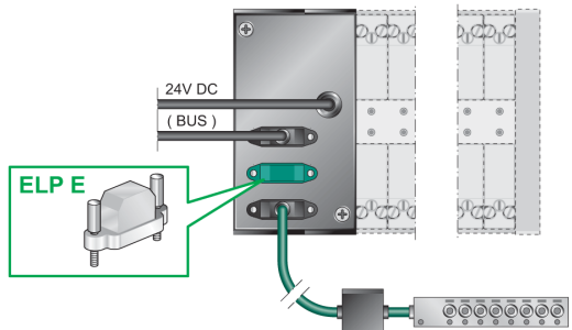
ELP I Wtyk zaślepiający do INPUT PORT
