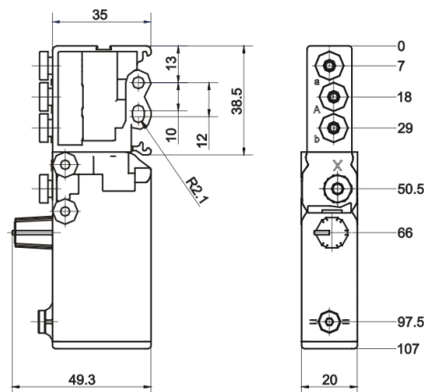
Maßzeichnung
