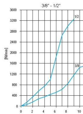
Obrati na vretenu
