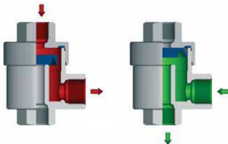
Smer protoka ka cilindru
