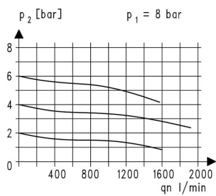
Durchflussdiagramm
