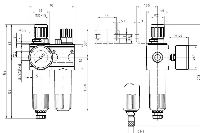
polavtomatski izpustni ventil
