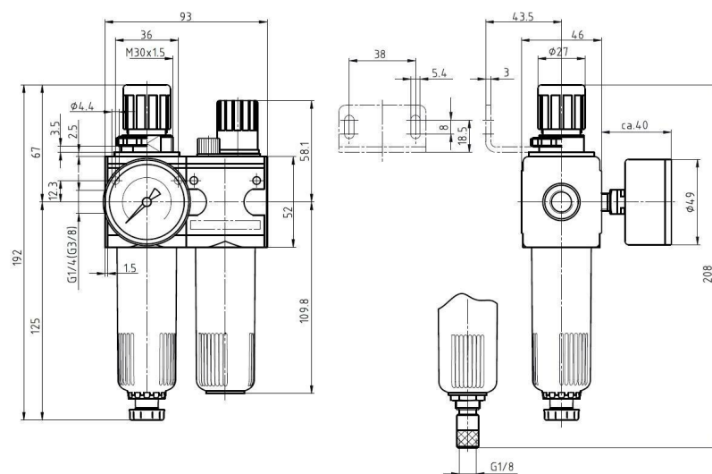
halbautomatisches Ablassventil
