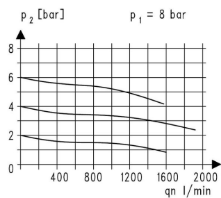
Durchflussdiagramm
