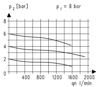
Átfolyási diagramm
