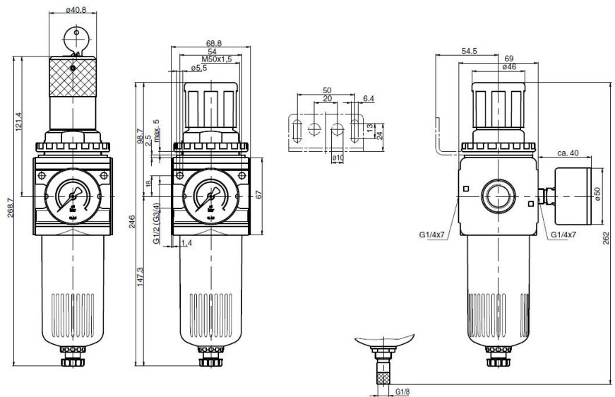
halbautomatisches Ablassventil
