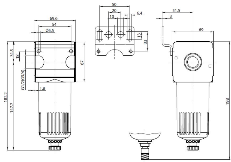
automatisches Ablassventil
