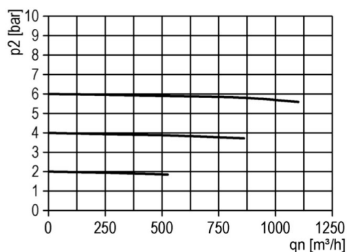
průtokový diagram
