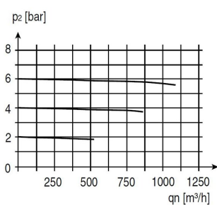
Průtokový diagramm
