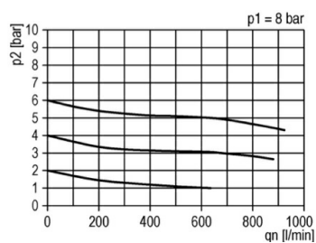
Průtokový diagramm
