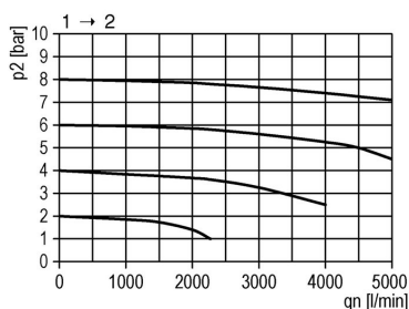
1. Átfolyási diagramm
