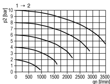
1. Átfolyási diagramm
