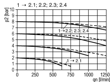
2. Wykres przepływu
