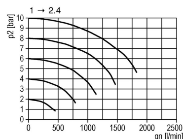
2. Dijagram protoka
