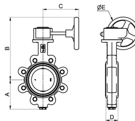
Abflanschausführung
