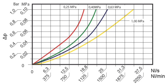
Wykres przedstawia różne ciśnienia wejściowe do spadku ciśnienia maks. 1bar
