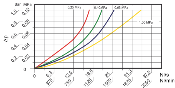
Dijagram prikazuje različite ulazne pritiske do pada pritiska maks. 1bar
