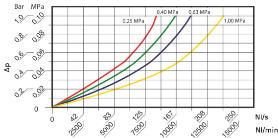
A diagram különböző bemeneti nyomásokat mutat legfeljebb 1 bar nyomásesésig
