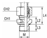
s řezným kroužkem B3
