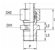
mit B3-Schneidring
