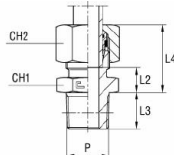
z pierścieniem tnącym B4
