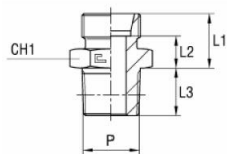
Osnovno telo
