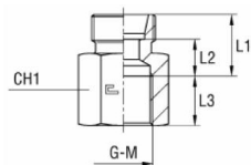
Základní těleso
